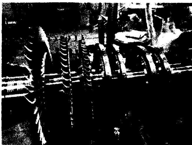
< 写真1 タービンローター >
